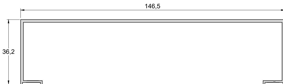
Guia de Persiana TL-046 0,937 kg/m
